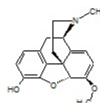
Oripavine
