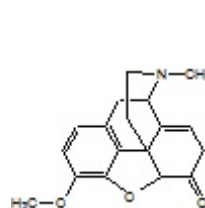
Neopinone
